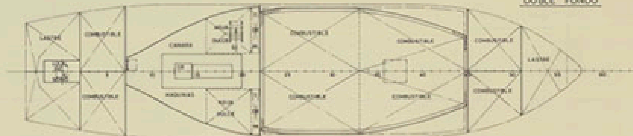
DOBLE FONDO
